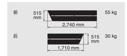
左侧通道总高度：150 mm
