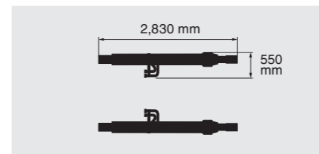
动臂油缸 550 kg×2 总高度：410 mm
